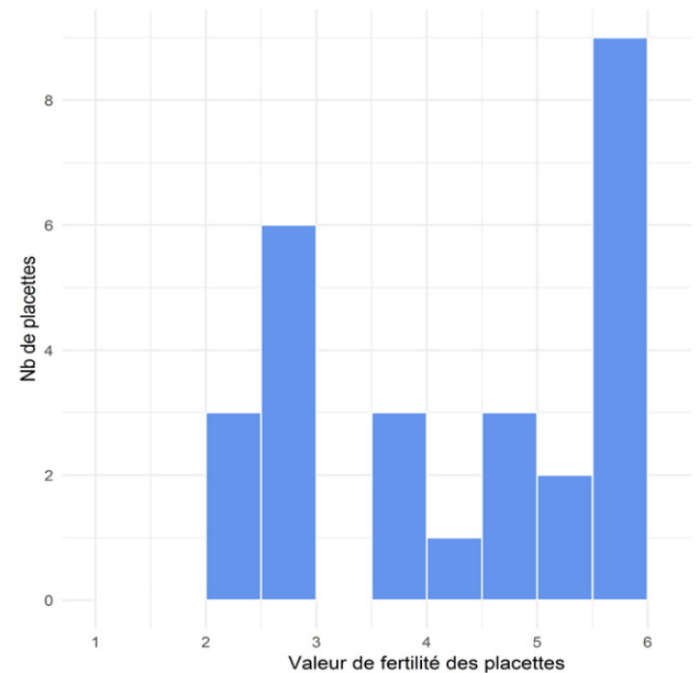
Figure 4 : valeur diagnostique de niveau de fertilité des placettes du site en 2017.
