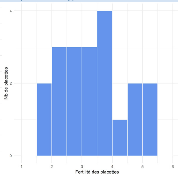
Figure 2 : valeur diagnostique de niveau de fertilité des placettes de type SDAGE 9 en 2017.
